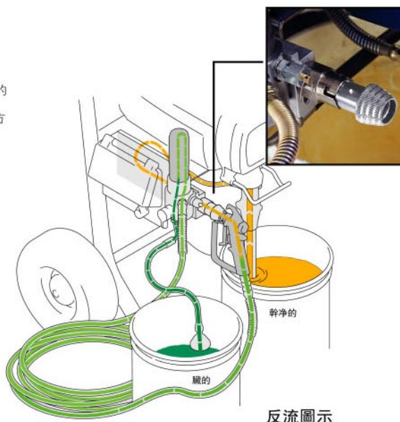
反流圖示
